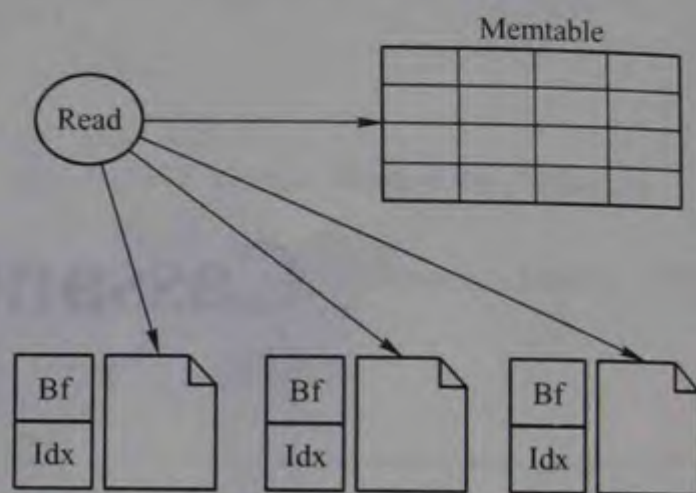
图 8-1 数据读取流程
