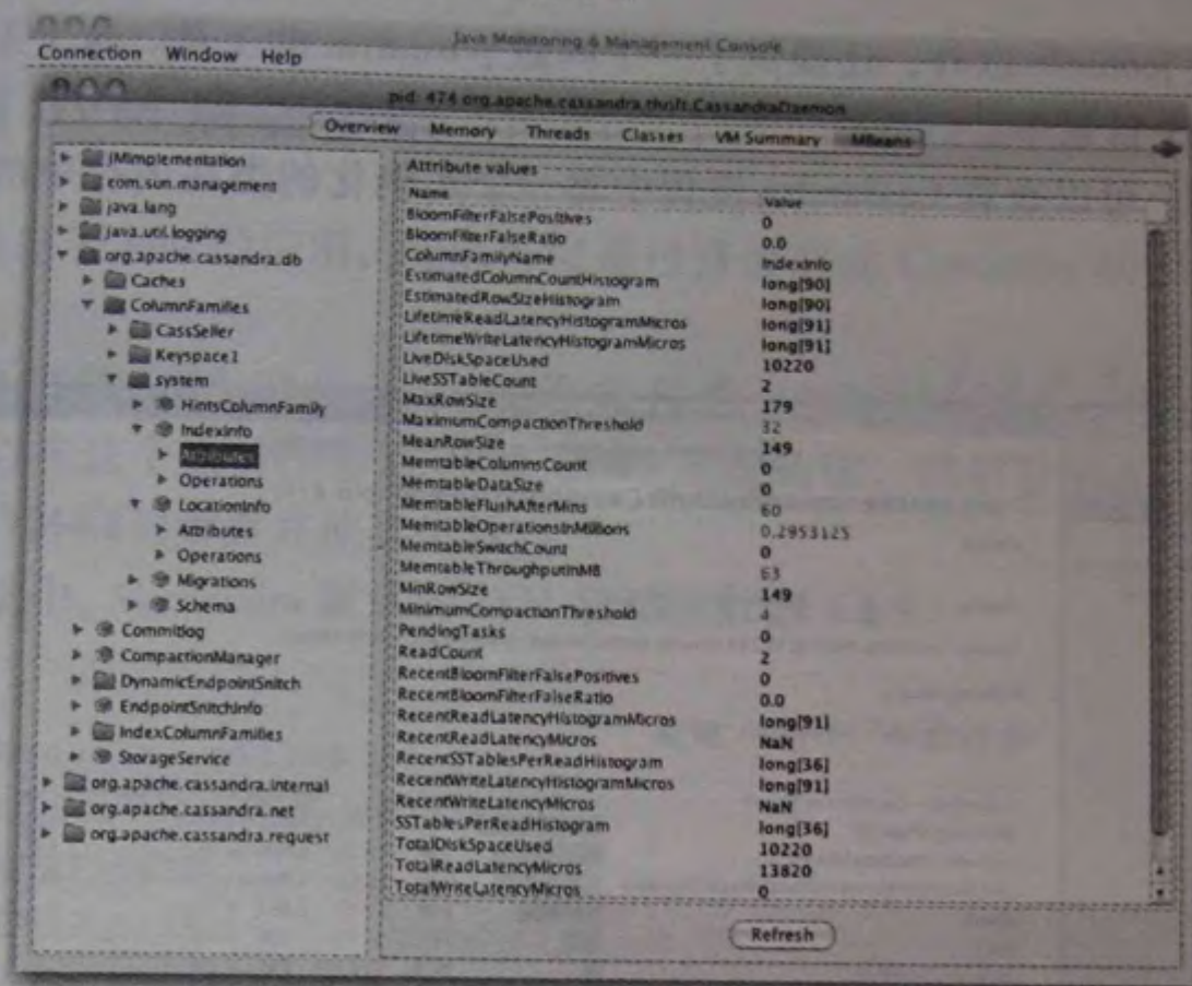
图 13-7 Cassandra 中的 JMX 变量的值
