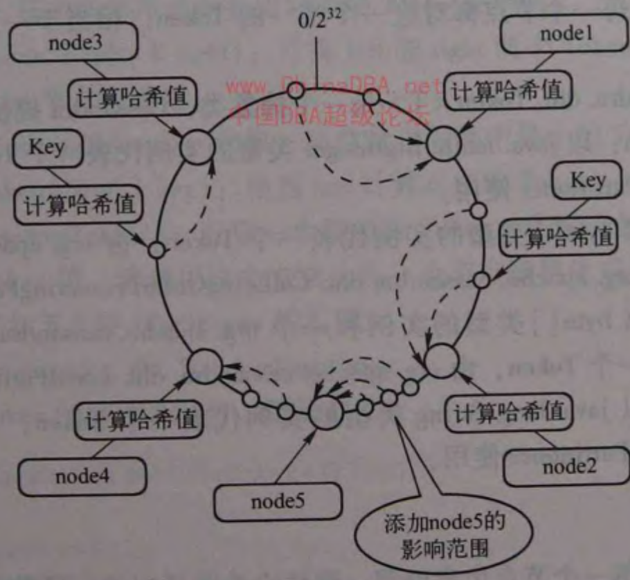
图 5-3 添加新的服务器
