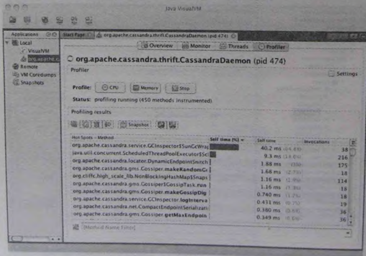
图 13-10 Cassandra 中方法调用次数和占用时间
