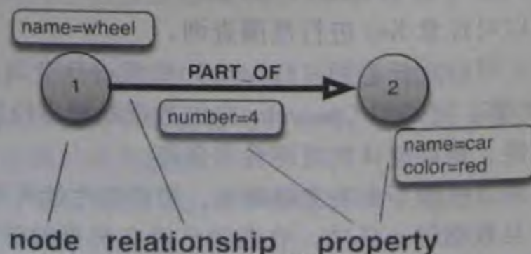
图 1-2 图模型的人元素示意图 www.ChinaDBA.net 中国DBA超级论坛
