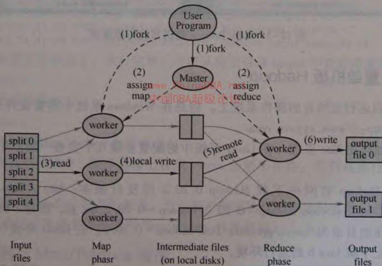
图 12-2 Map/Reduce 执行流程图
