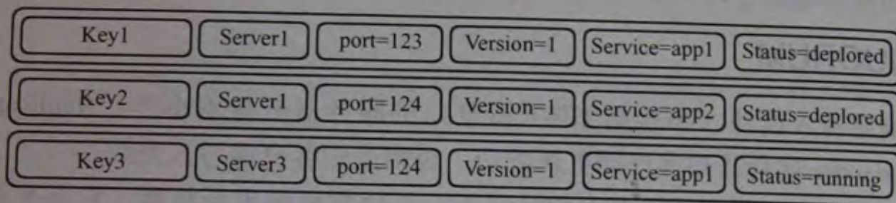
图 7-2 数据模型 1
