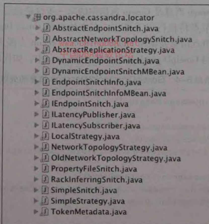
图 5-6 org.apache.cassandra.locator 代码结构
