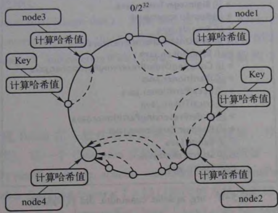
图 5-2 一致性哈希示意图
