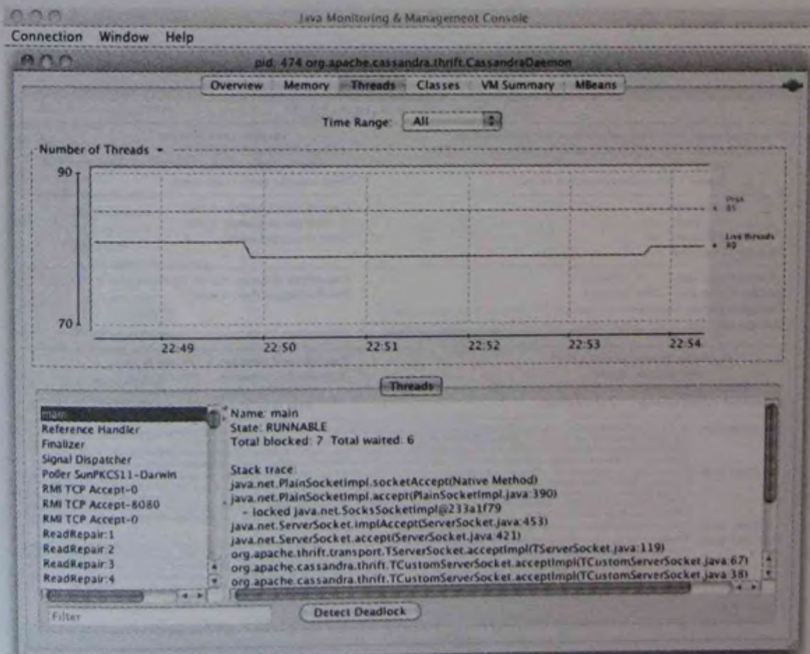
图 13-4 Cassandra 线程工作情况
