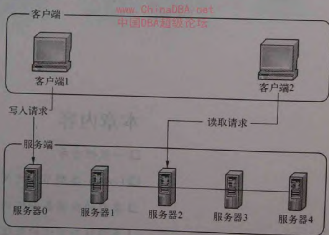
图 5-1 简单集群结构图
