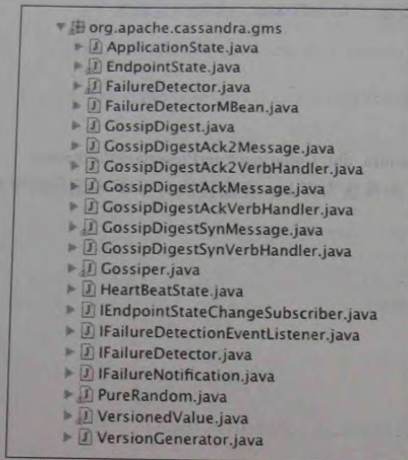
图 5-5 org.apache.cassandra.gms 代码结构 中国DBA超级论坛
