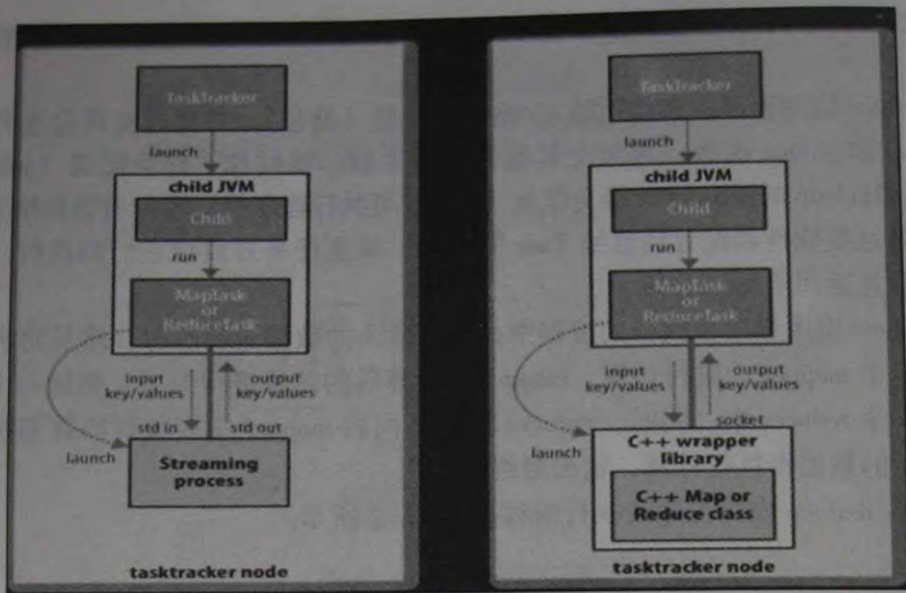
图 12-3 Map/Reduce 跨语言执行原理图
