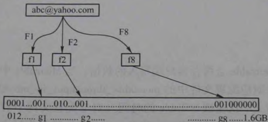
图 6-1 布隆过滤器示意图
