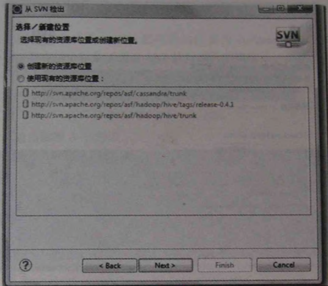
www.ChinaDBA.net 图 A-4 创建新的资源库位置
